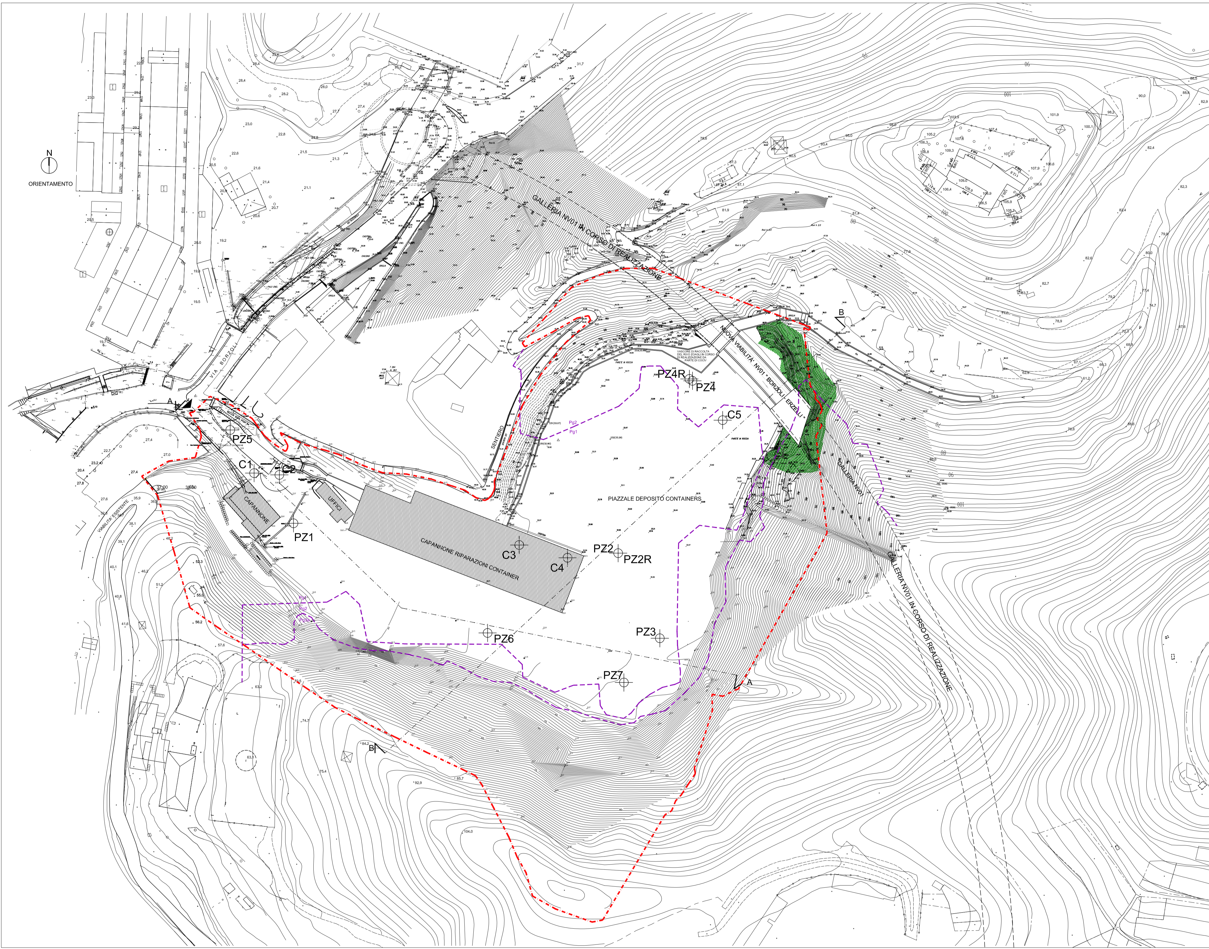
1 Planimetria Generale Rilievo Stato di Fatto 1/1000
